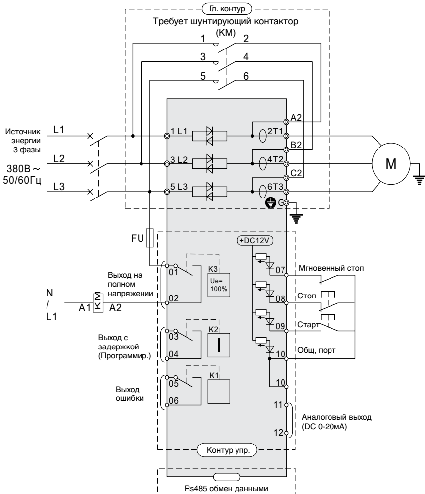
Рисунок 2-3-1 Схема подключения
