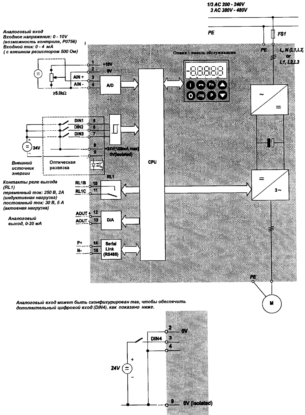
Рис. 3-7 Блок-схема преобразователя
